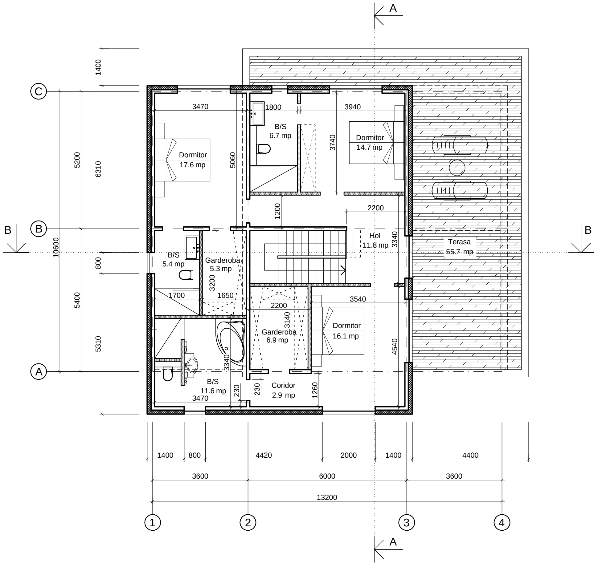
Plan etaj 1 Cota 3.600, Sc 1:100
